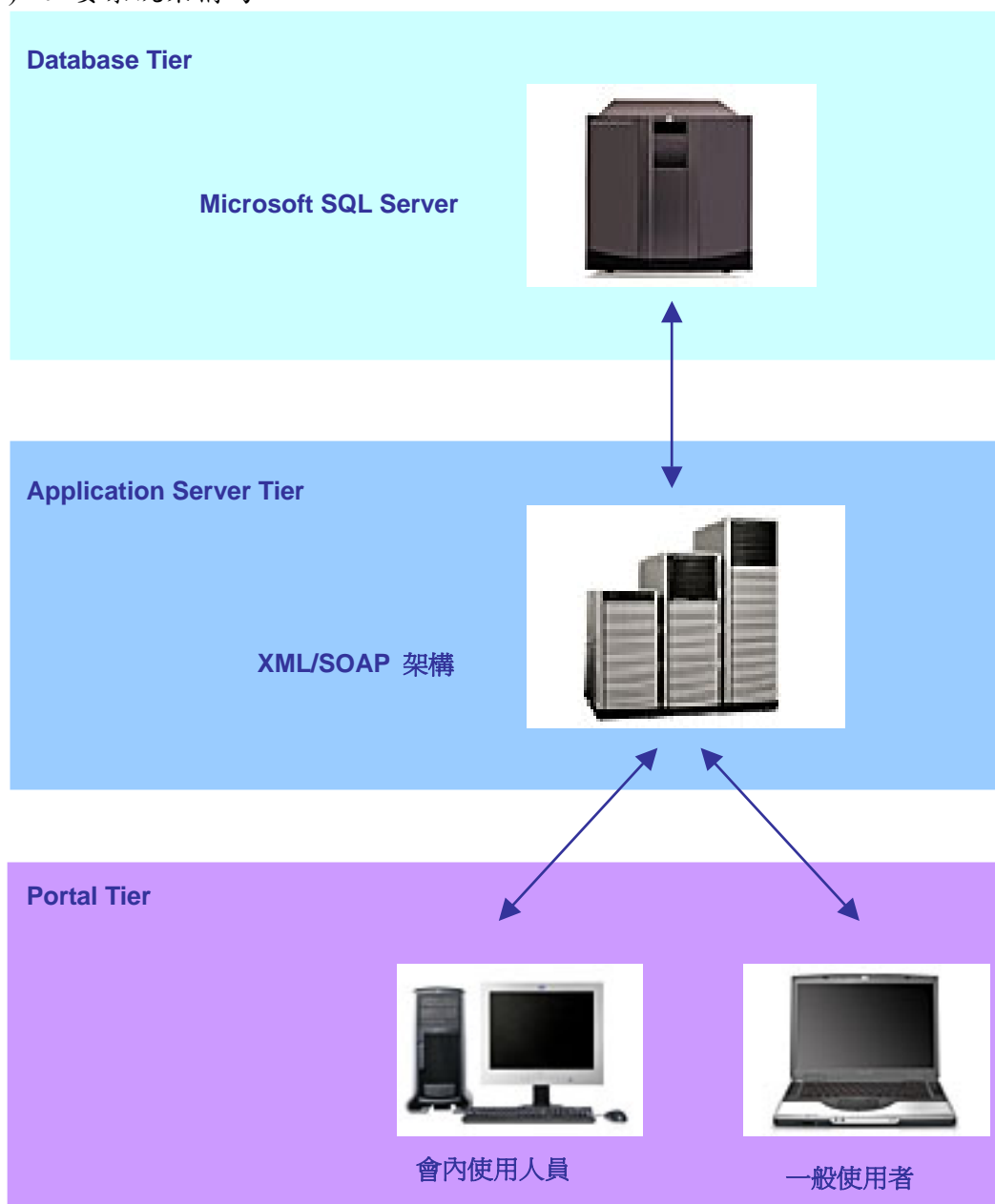
圖 4 台灣原住民族文化影音資料庫架構圖
