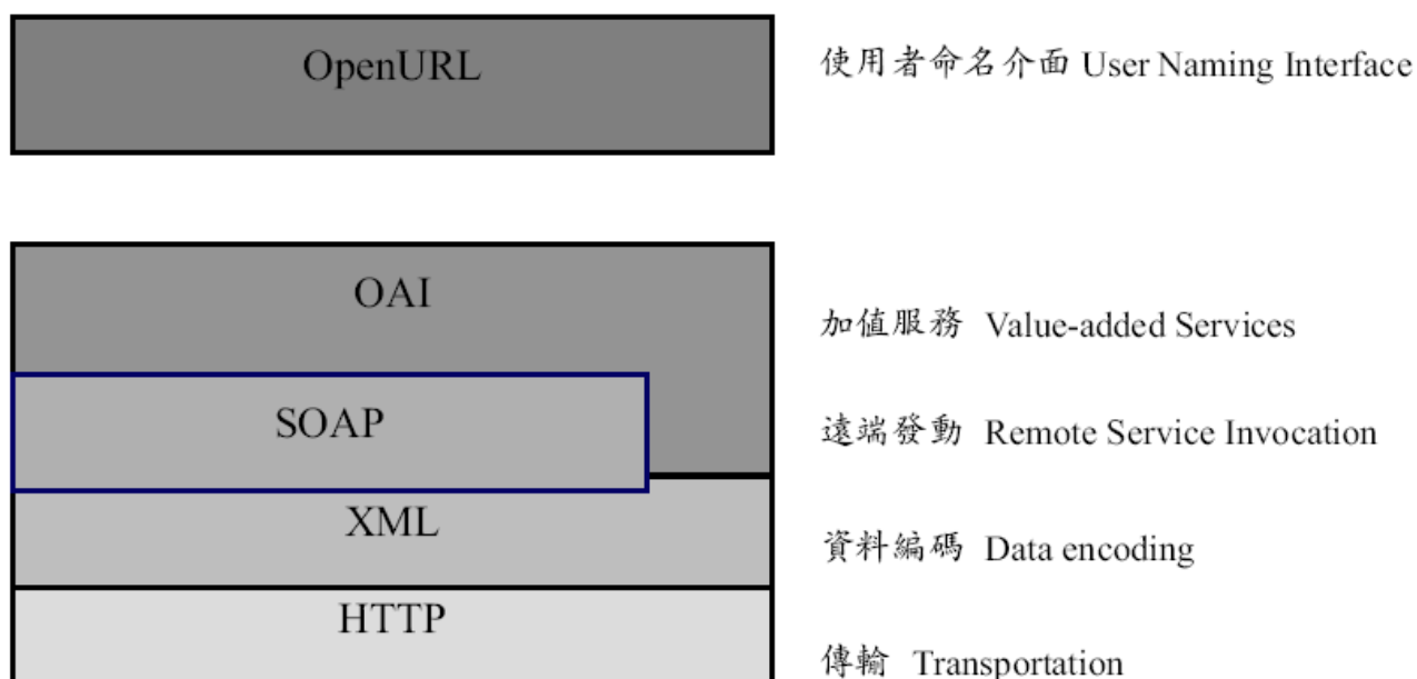
圖 16 各通信協定整合示意圖
