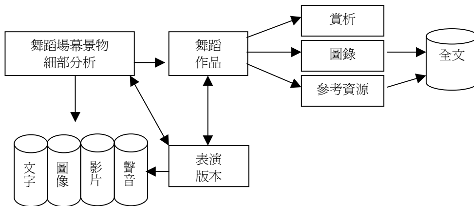
圖 20 舞蹈之 Metadata Model
