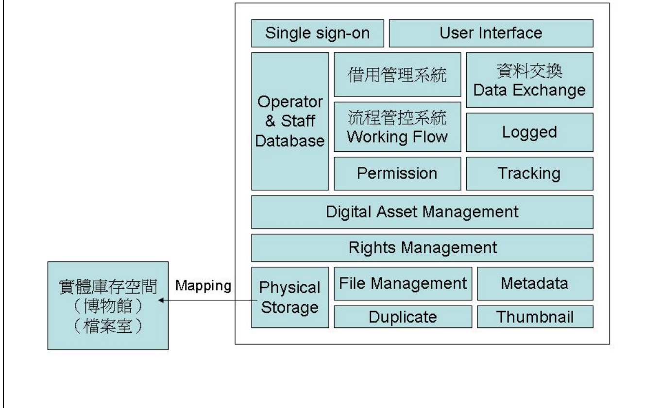
圖 2 典藏管理系統架構圖
