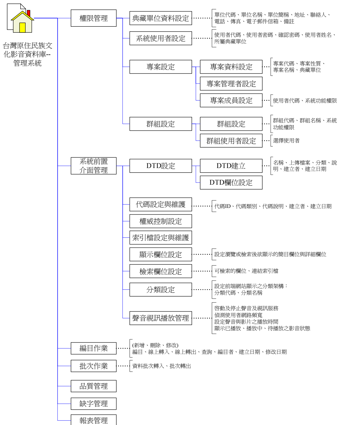
圖 6 台灣原住民族文化影音資料庫後端管理系統架構
