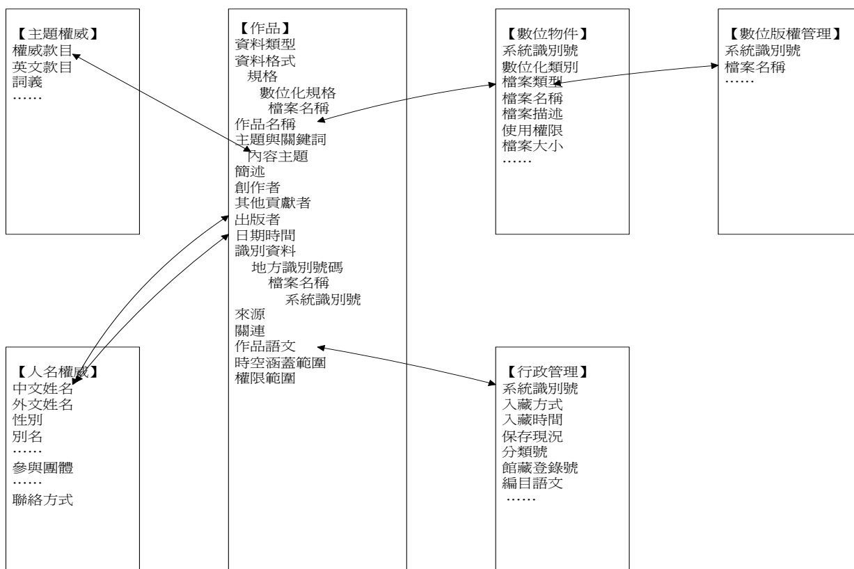
圖 25 數表結合模式範例二
