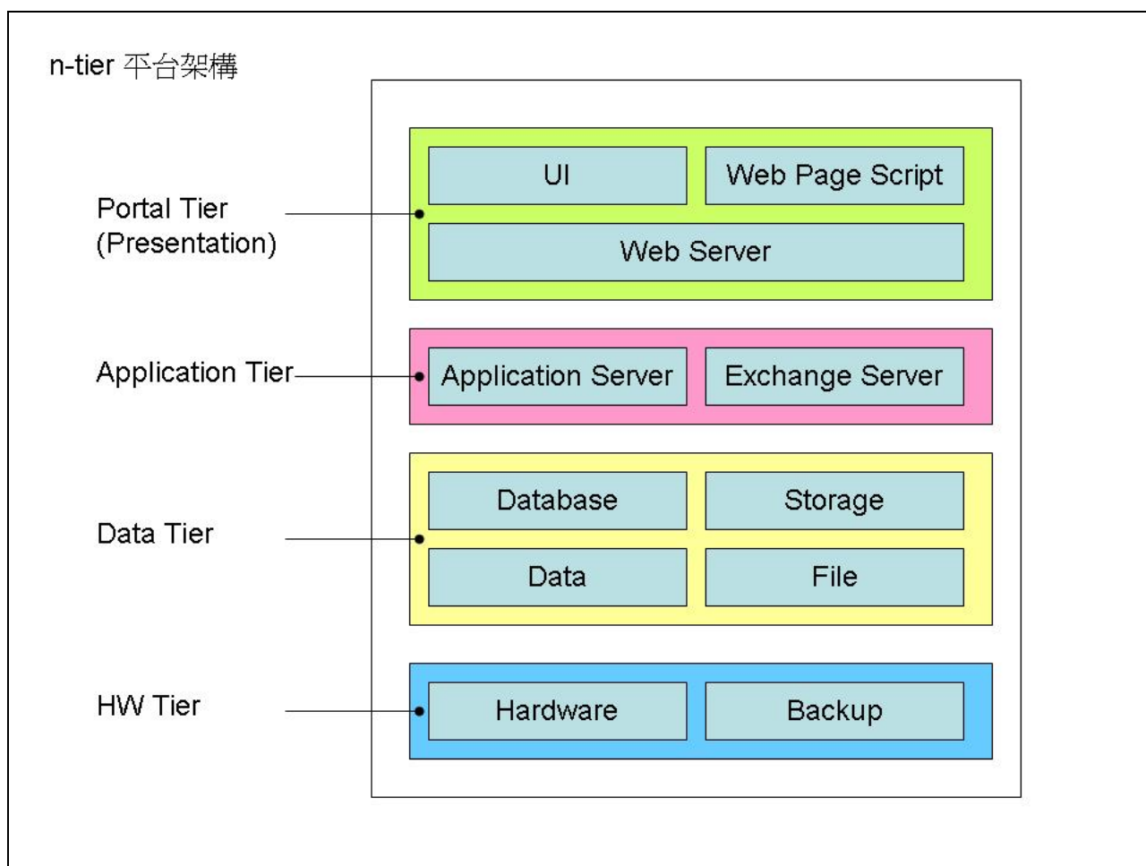
圖 3 n-tier 多層次架構概念圖
