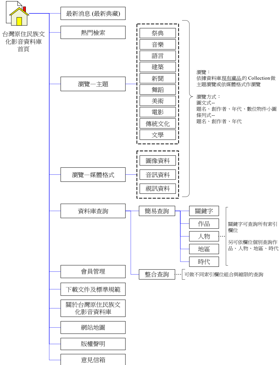
圖 5 台灣原住民族文化影音資料庫前端網站架構
