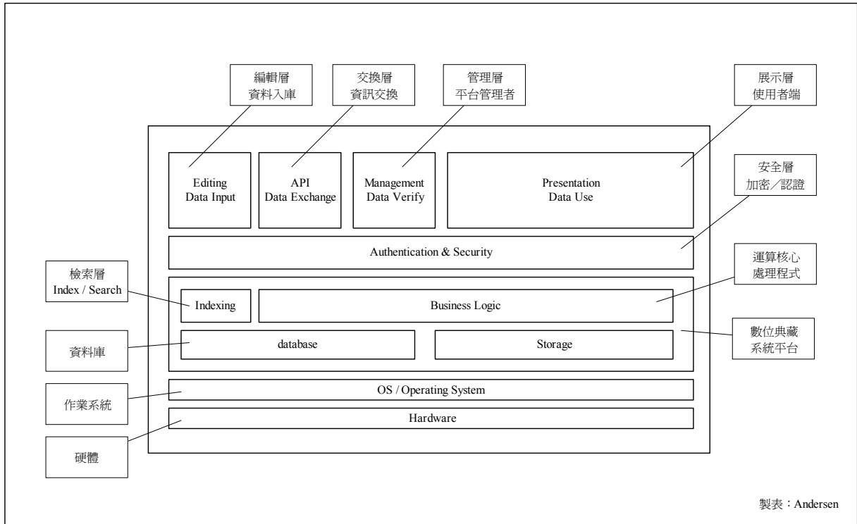
圖 13 n-tier 多層次互動架構
