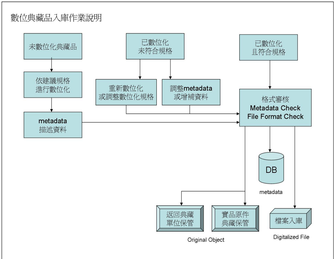
圖 19 數位典藏品入庫作業說明
