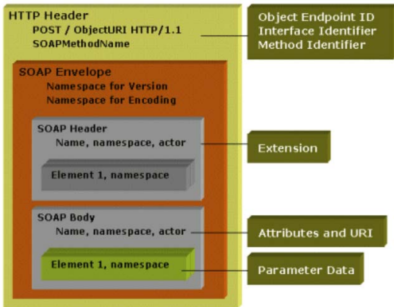
圖 18 標準 SOAP 訊息結構
