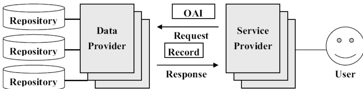
圖 17 OAI 結構示意圖
