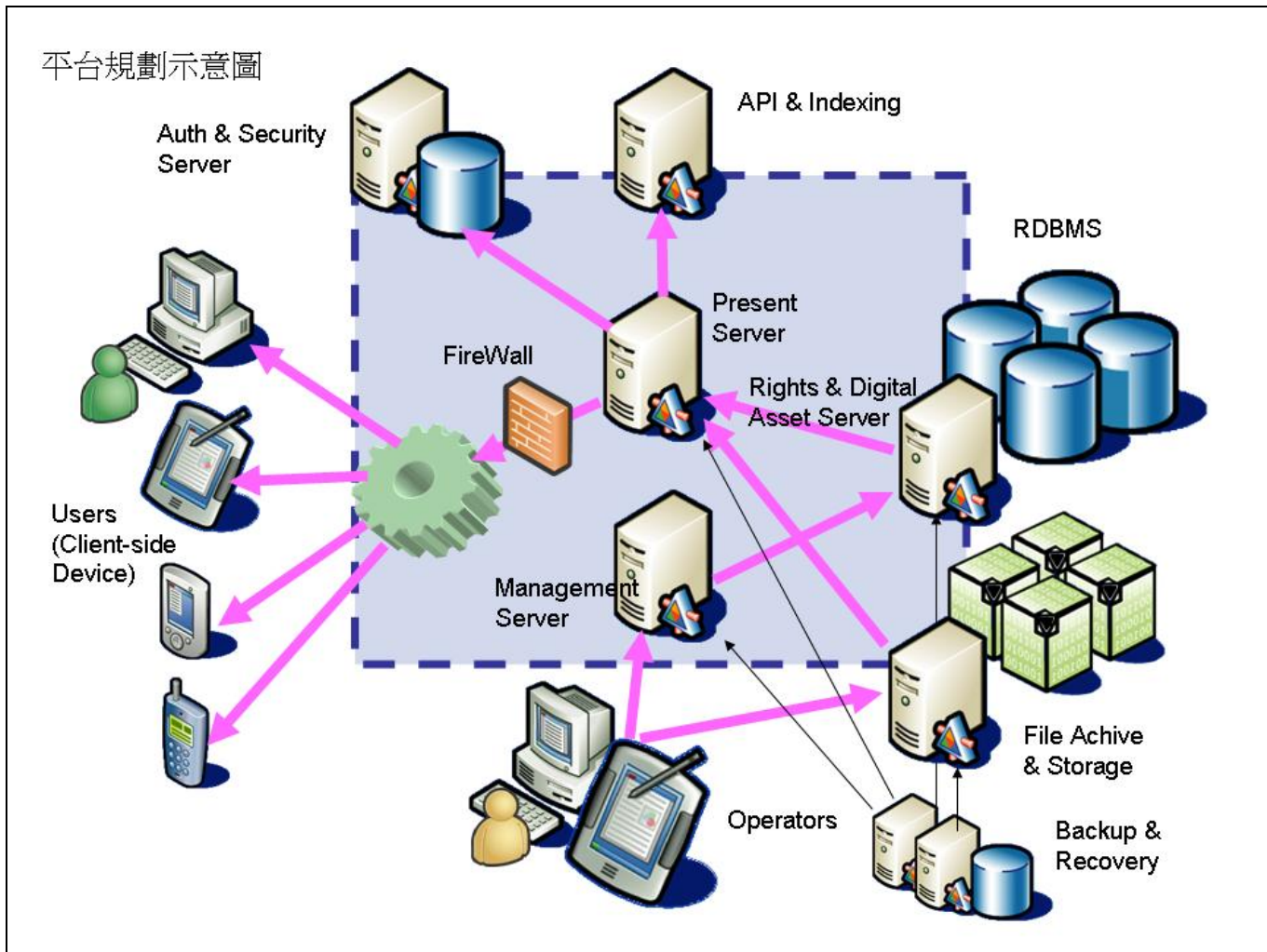
圖 15 平台規劃示意圖
